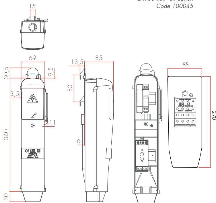
Borne de terre 2 x 35 mm 2 en option Code 100045
